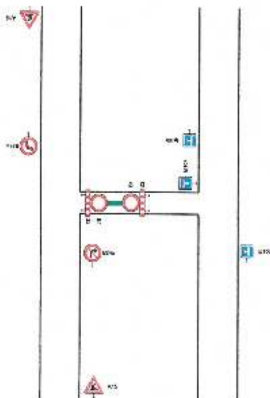
Schema 4. podélný výkop (stezá ulice) úplná uzavírka ulice
